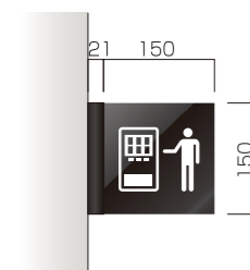
FBY-150 突出 標準価格 ¥14,700(外税)
