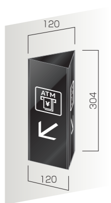
FBP-30 表示寸法 W100×H300 標準価格 ¥20,000(外税)
